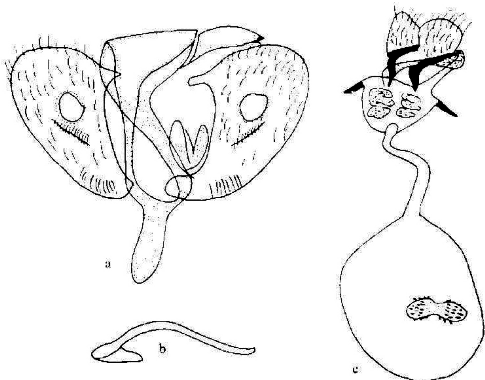
图 106 大翅绢粉蝶 Aporia largeteau (Oberthür)
